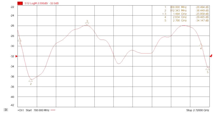
【图2】隔离度 Isolation
