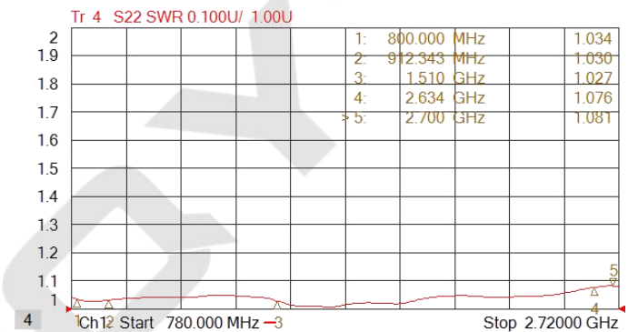
【图4】分配端驻波比Output Port VSWR
